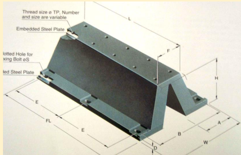
รูปที่ 2 ยางกันกระแทกรูปตัว V
