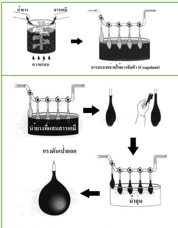
รูปที่ 1 ตัวอย่างกระบวนการผลิตลูกโป่ง
