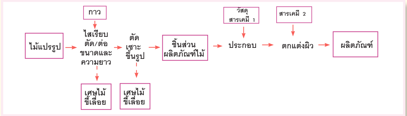
รูปที่ 1 กระบวนการผลิตเฟอร์นิเจอร์และผลิตภัณฑ์ไม้
